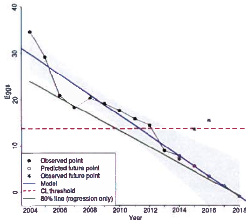
Regression - 2004 - 2013 eden
