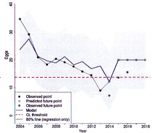
MA - 2004 - 2013 eden
