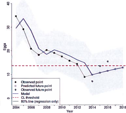
AR - 2004 - 2013 eden
